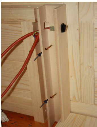
Fig. 33: Montagem das barras em U para pacas de aquecimento
