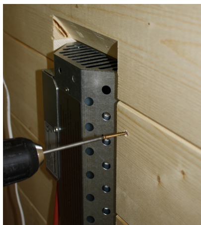
Fig. 39: Montar o painel dos radiadores traseiros
