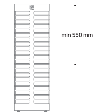
Рисунок 2. Установка каменки HUUM STEEL, частично погруженной в потолок.
