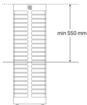
Kuva 2. HUUM STEEL sähkökiukaan upotus lauteisiin
