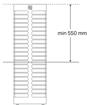
Figur 2. HUUM STEEL bastuugnens montering i svettbänken
