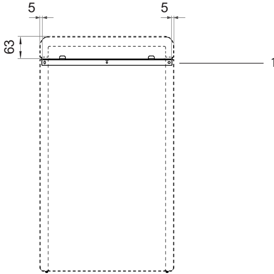
Kuva 3 Concept R mini -asennuslistan paikka Mittayksikkö mm
