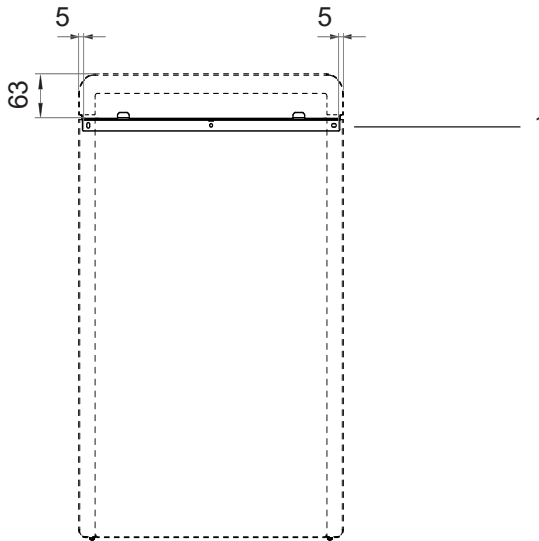
Bild 3 Positionering av monteringslist Concept R mini mått i mm
