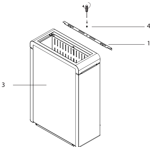
Fig. 4 Fixation du Concept R mini (barre de montage)
