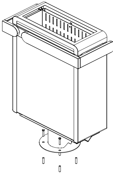
Fig. 6 Fixation du Concept R mini avec pied
