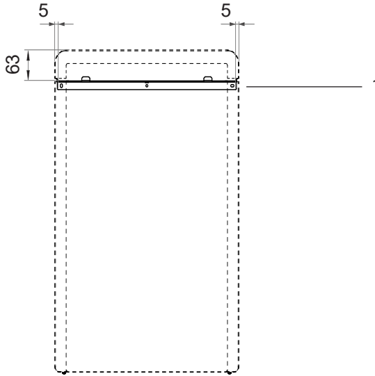
Abb.3 Position der Montageleiste Concept R mini Maße in mm
