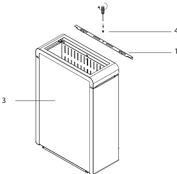
Fig. 4 Fissaggio di sicurezza Concept R mini (listello di montaggio)
