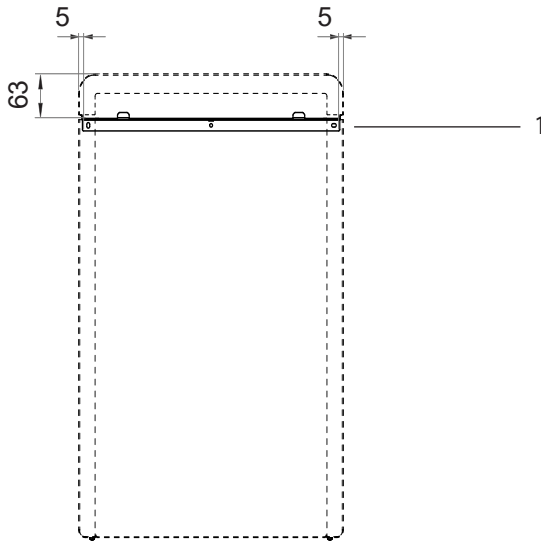
afb. 3 Positie van de montagelijst Concept R mini afmetingen in mm
