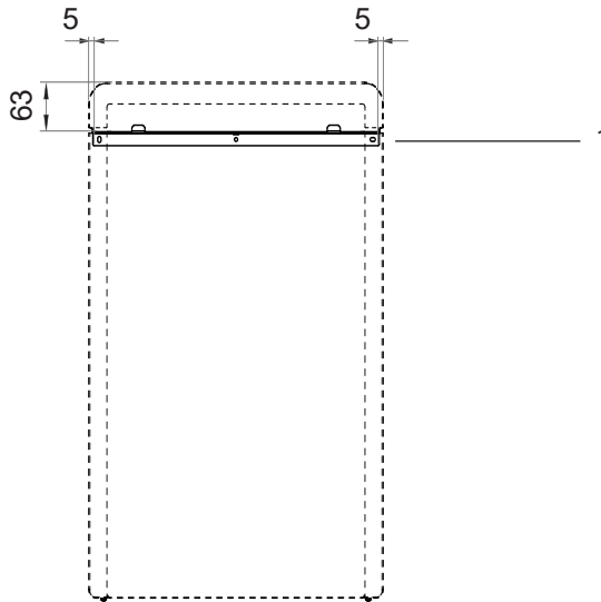
Fig. 3 Posizione del listello di montaggio Concept R mini Dimensioni in mm
