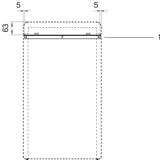
Fig. 3 Position de la barre de montage du Concept R mini Dimensions en mm
