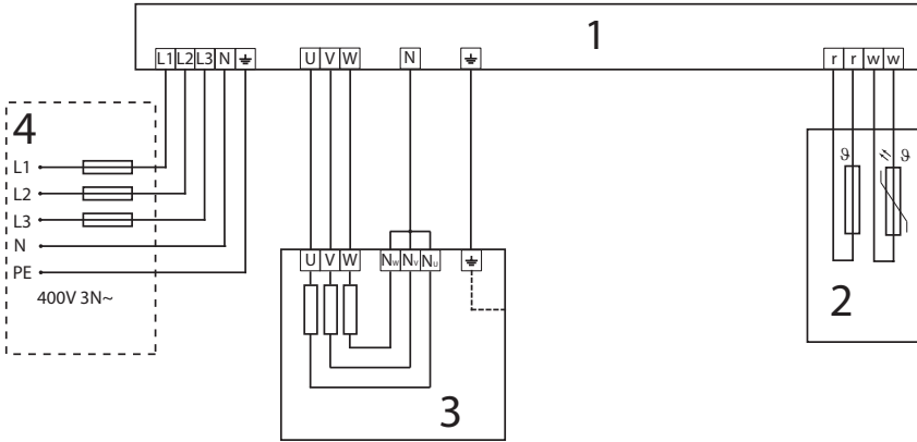
Abb.8 Anschlussplan Concept R mini 3,5 kW, 4,5 kW, 6,0 kW und 7,5 kW (CP-RM-35 / CP-RM-45 / CR-RM-60 / CP-RM-75)
