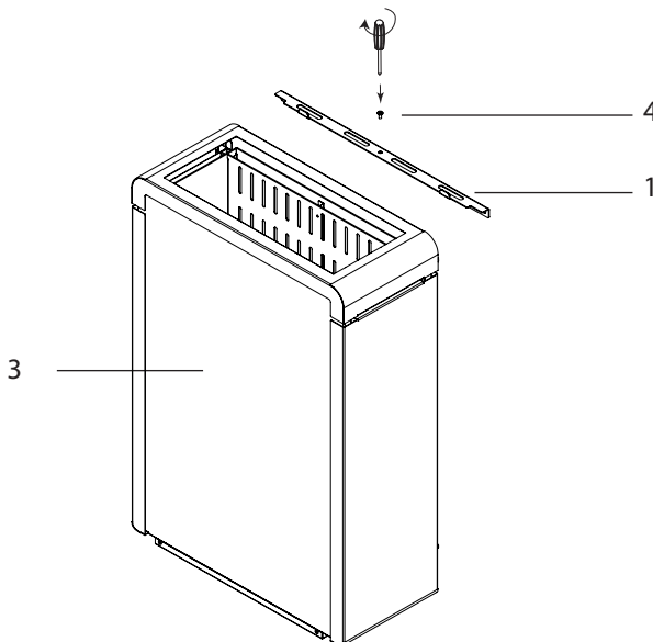
Bild 4 Fastsättning Concept R mini (monteringslist)
