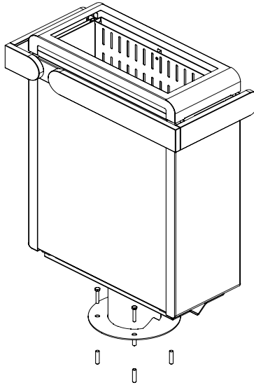
Abb.6 Fixierung Concept R mini mit Standfuß
