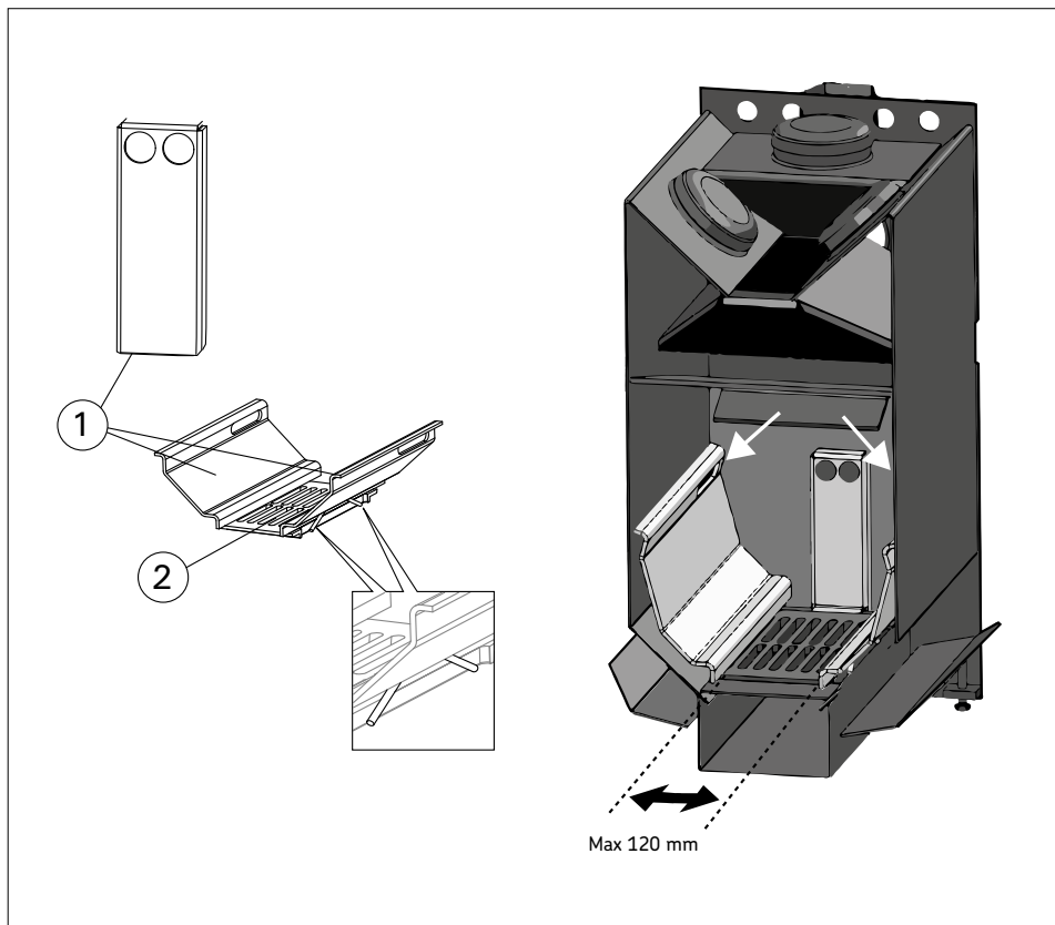
Kuva 2. Palamisilmanohjaimet.
