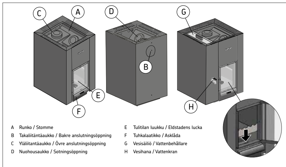
Kuva 1. Kiukaan osat.
