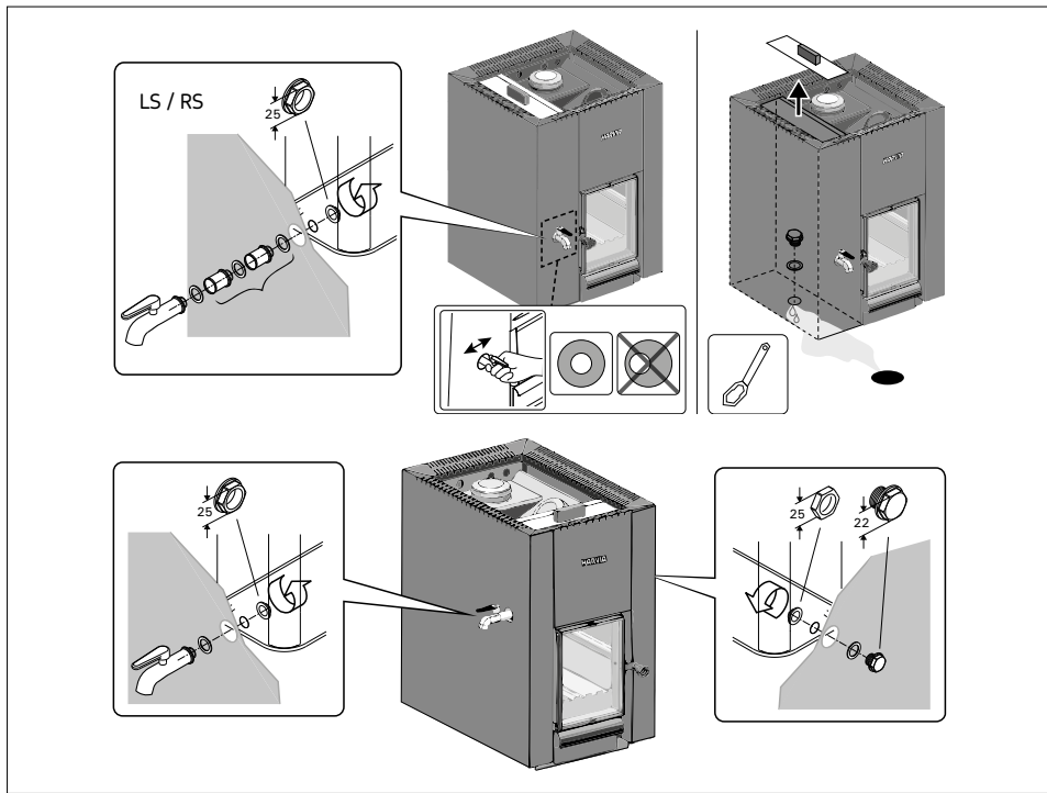
Kuva 3. Vesihanau asennus. Bild 3. Montering av vattenkran.
